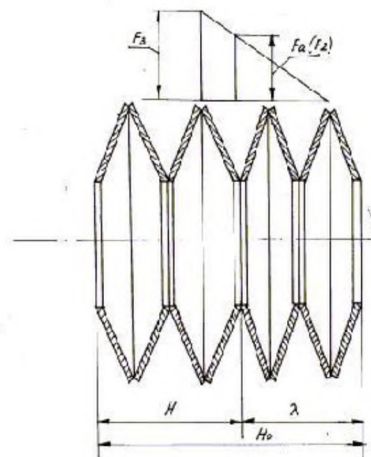
Рис. 15.2.3 Расчетные размеры
