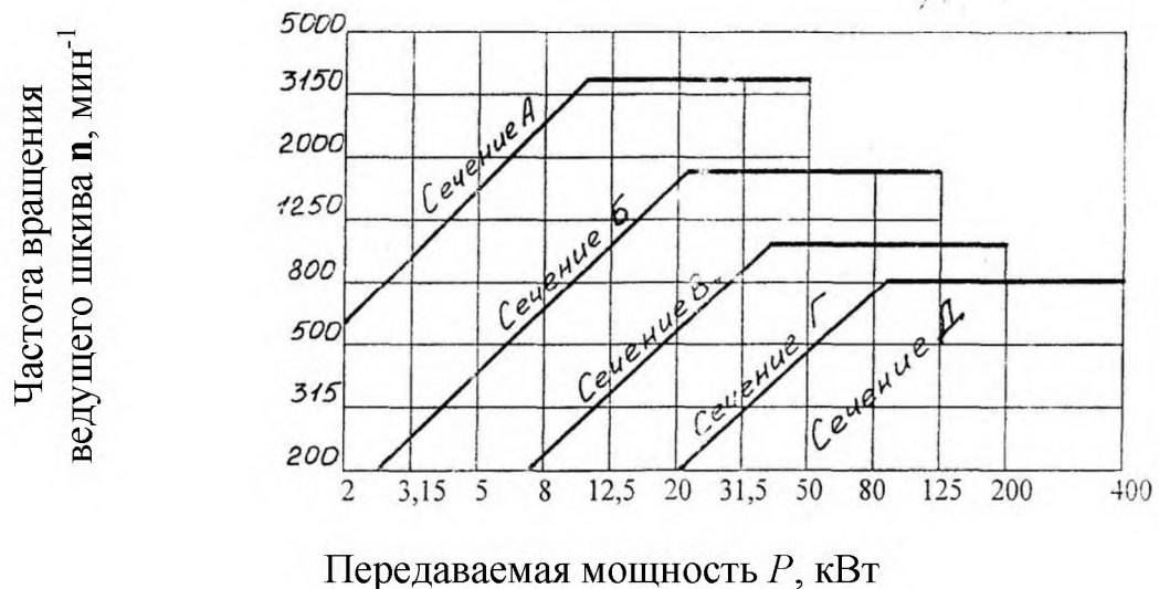
Рис. 3.1.3 Номограмма для выбора сечения клинового ремня рассчитываемой передачи
