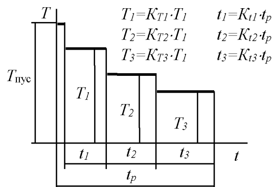
Рис. 1.2 Циклограмма нагружения
