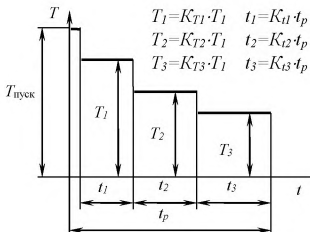
Рис. 3.1.2 Циклограмма нагружения
