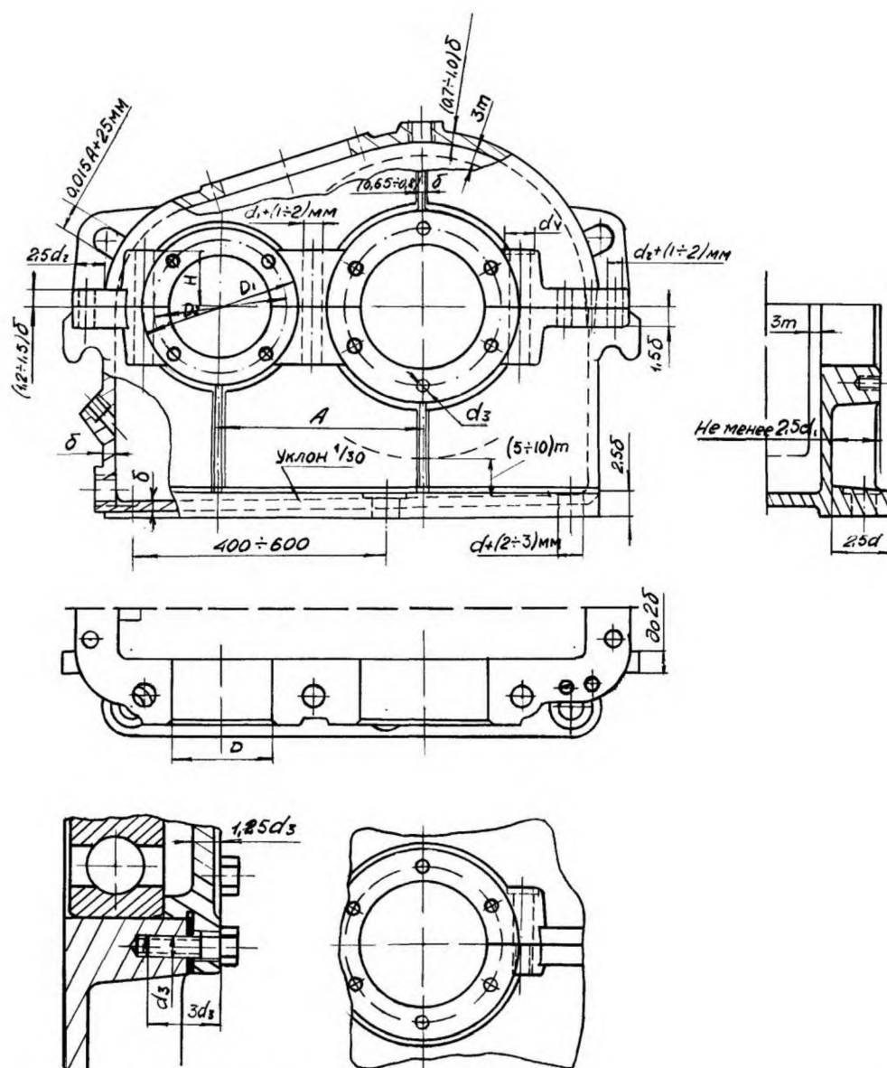
Крепление крышки подшипника
